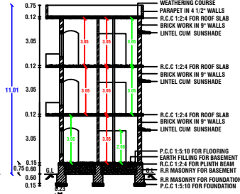
SECTION A-B
