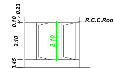
ELEVATION
