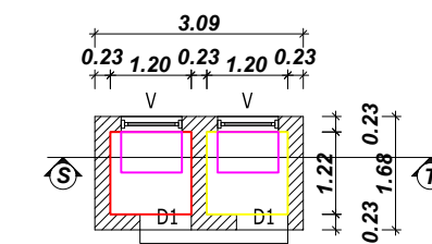
TOILET PLAN
