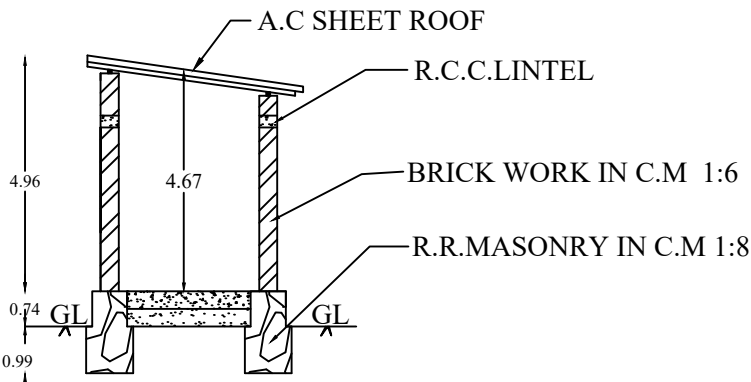
TOILET SECTION
