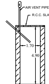
SOAK PIT
