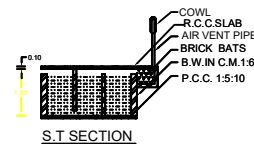
S.T SECTION
