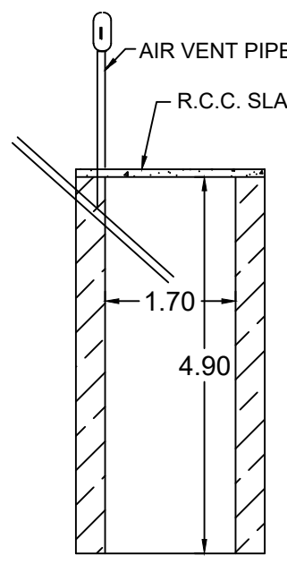
SOAK PIT
