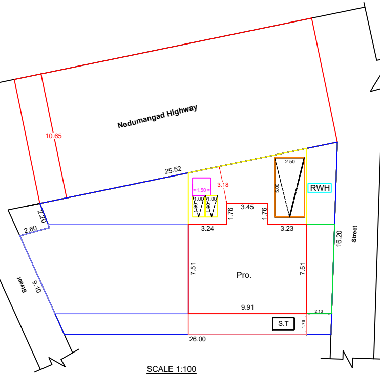
SCALE 1:100 SITE PLAN
