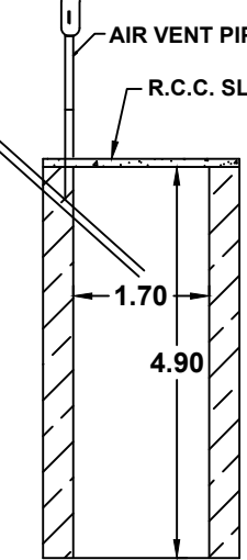
SOAK PIT
