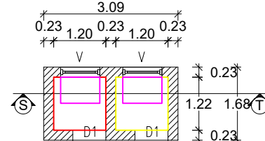
TOILET PLAN
