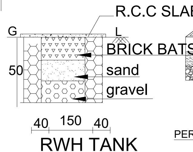
R.W.H. TANK
