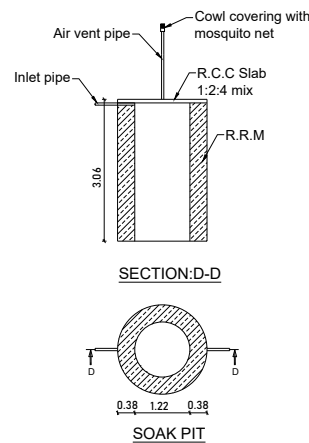
SOAK PIT
