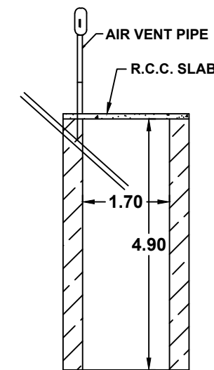
SOAK PIT
