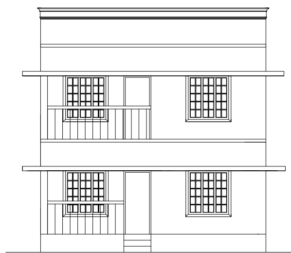
ELEVATION
