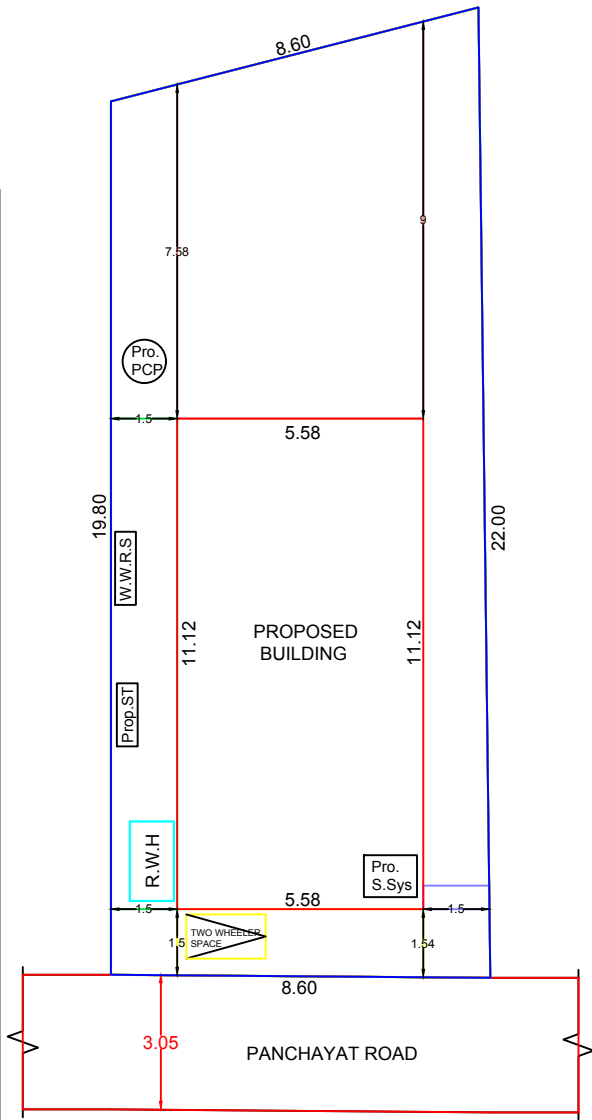
SITE PLAN 1:100
