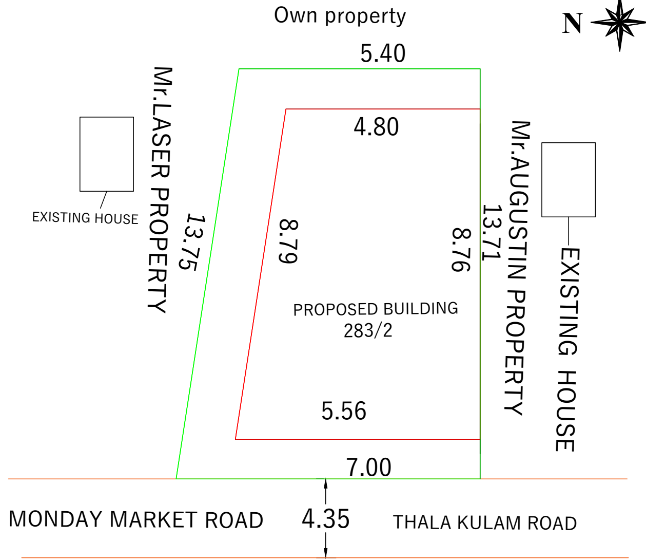
KEY PLAN SCALE : NIL
