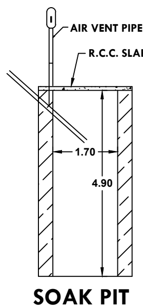
SOAK PIT
