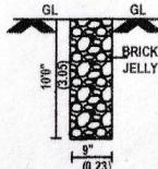
LONGITUDINAL SECTION
