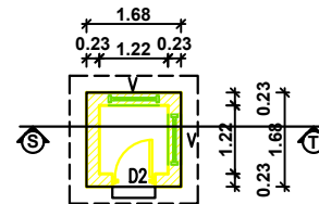
TOILET PLAN
