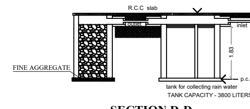
SECTION D-D
