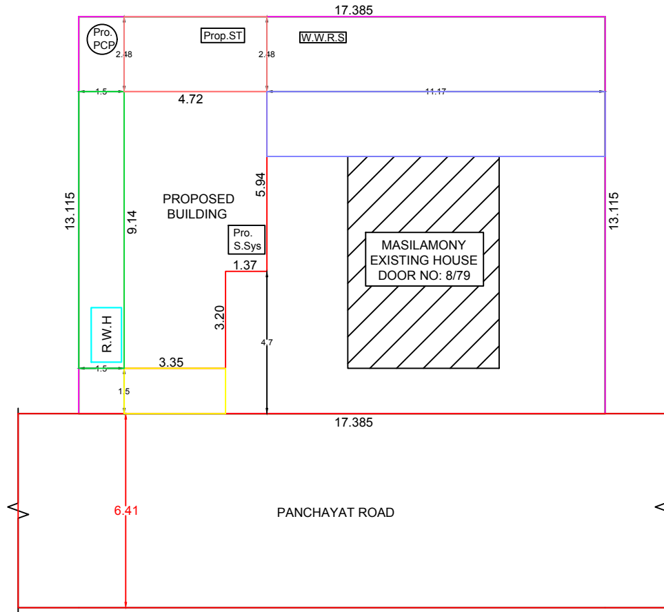
SITE PLAN 1:100
