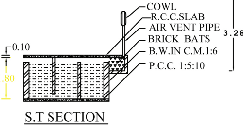
S.T SECTION
