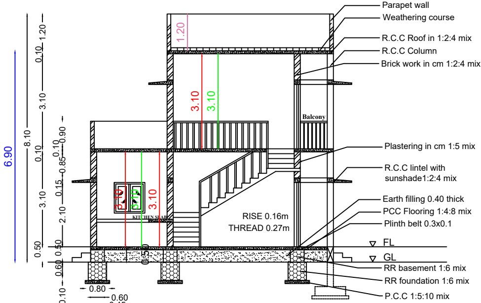
SECTION -AB
