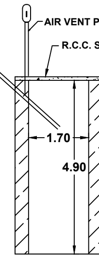
SOAK PIT
