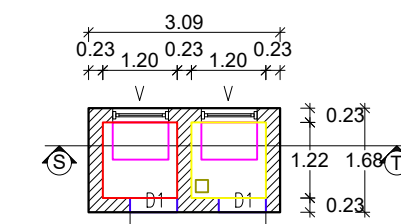
TOILET PLAN
