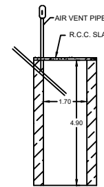
SOAK PIT
