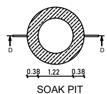
SOAK PIT
