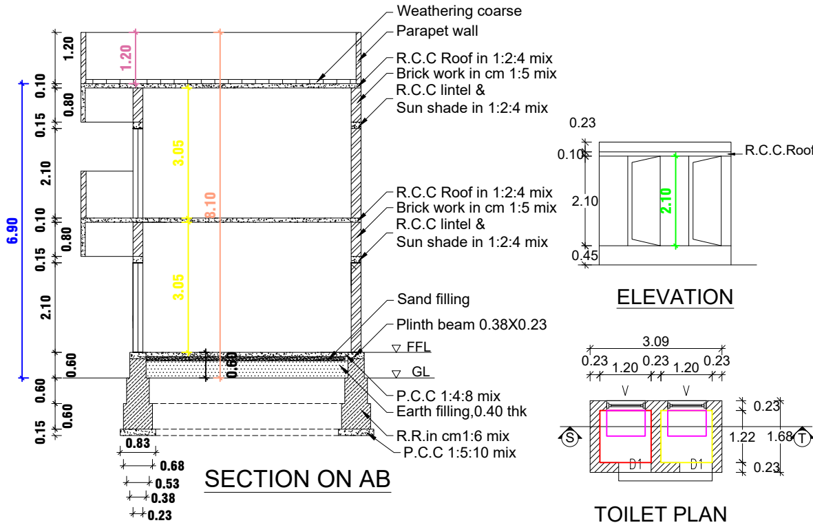
TOILET PLAN
