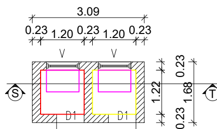
TOILET PLAN
