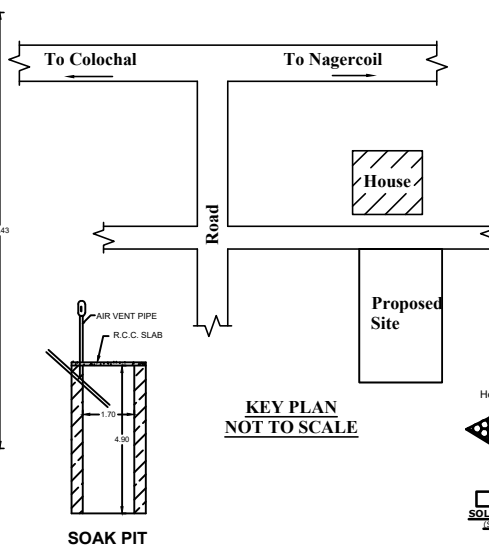
SOAK PIT
