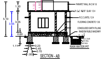
SECTION - AB
