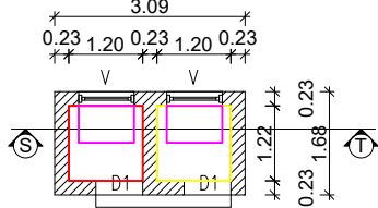
TOILET PLAN
