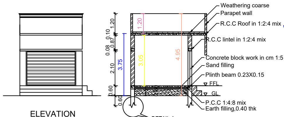
ELEVATION
