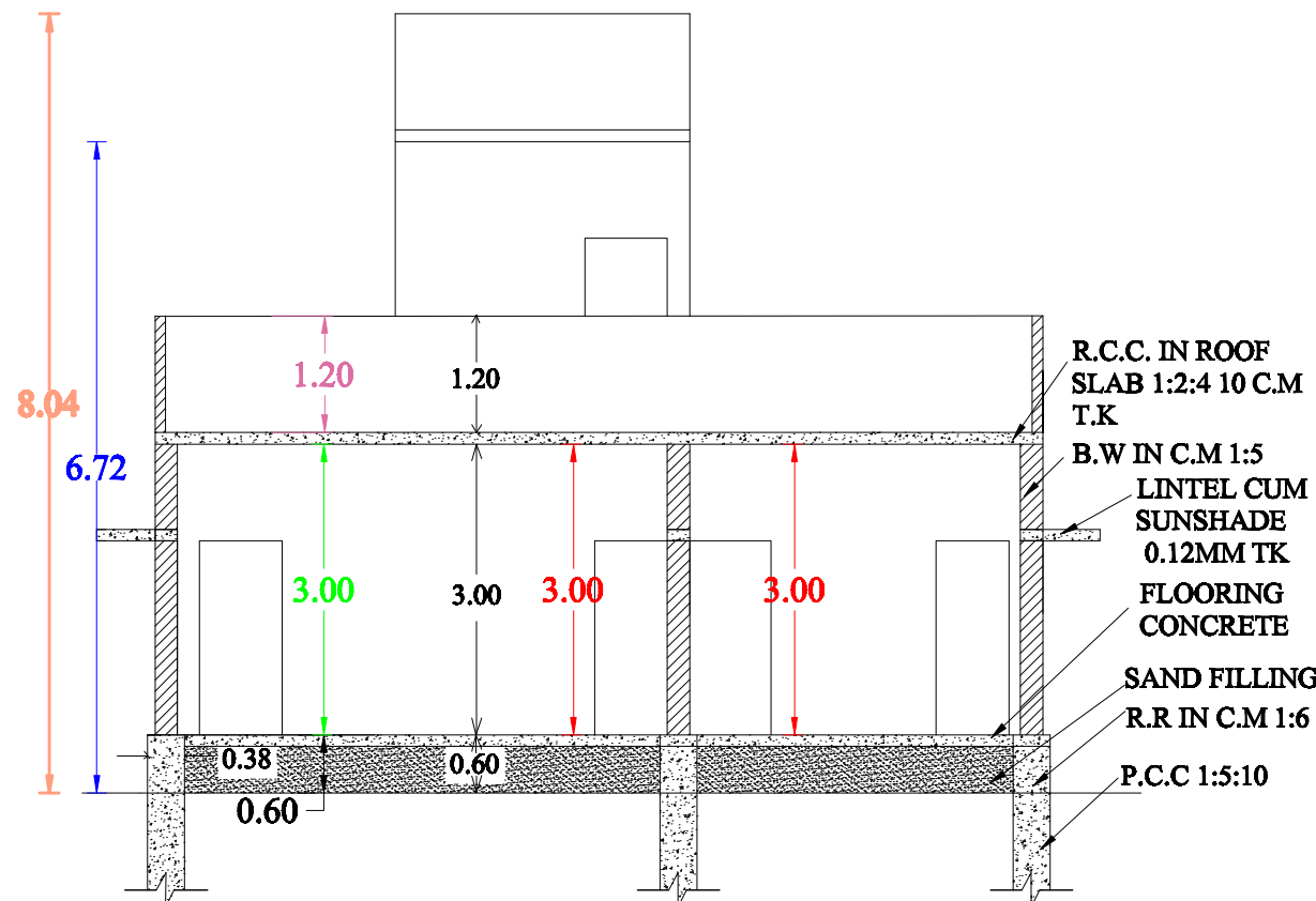
SECTION A-B
