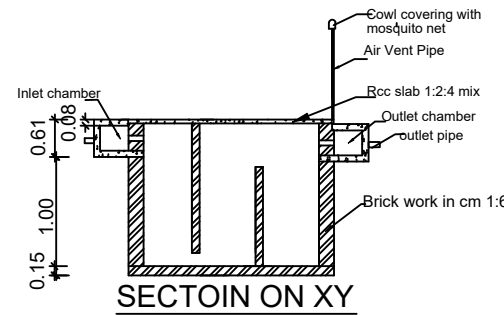
SECTOIN ON XY
