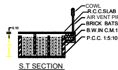
S.T. SECTION
