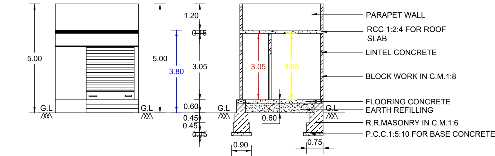
ELEVATION
