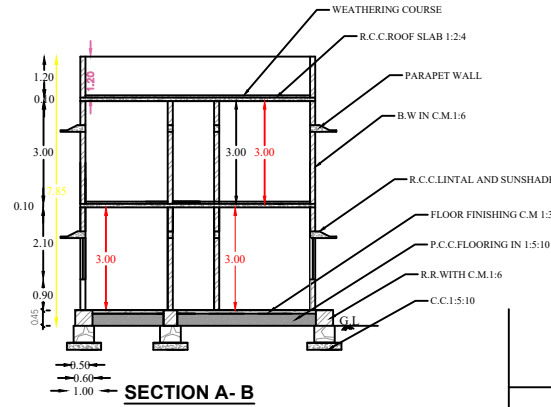
SECTION A-B
