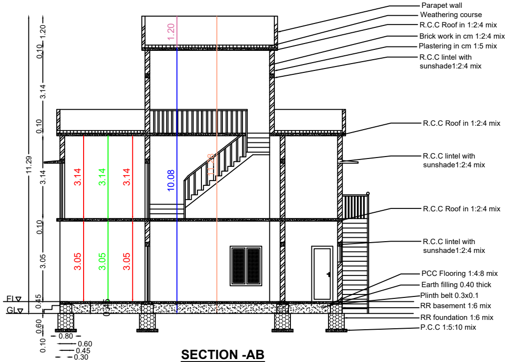
SECTION -AB
