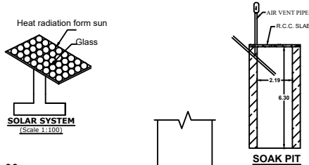
SOAK PIT
