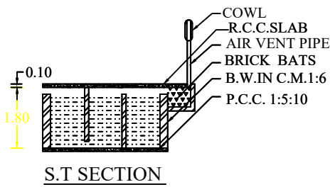
S.T SECTION
