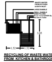
SOAK PIT
