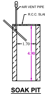
SOAK PIT
