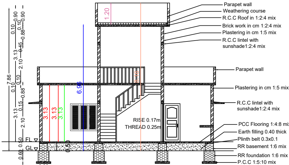
SECTION -AB
