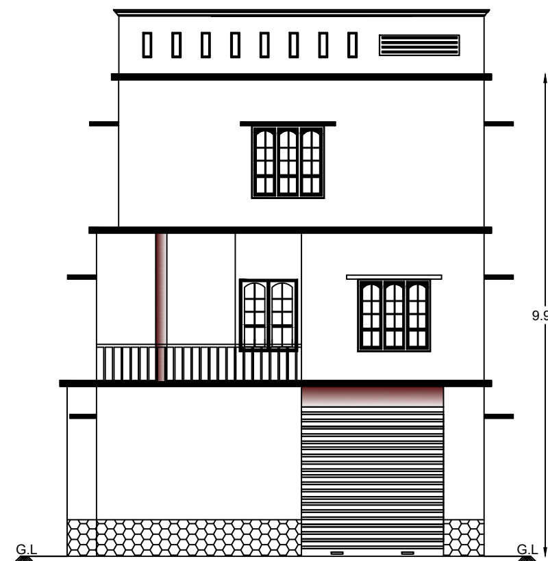
ELEVATION
