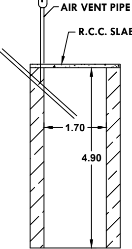
SOAK PIT
