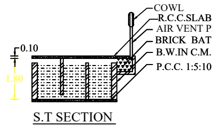
S.T SECTION
