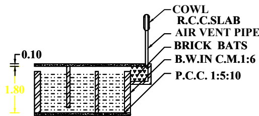
S.T. SECTION
