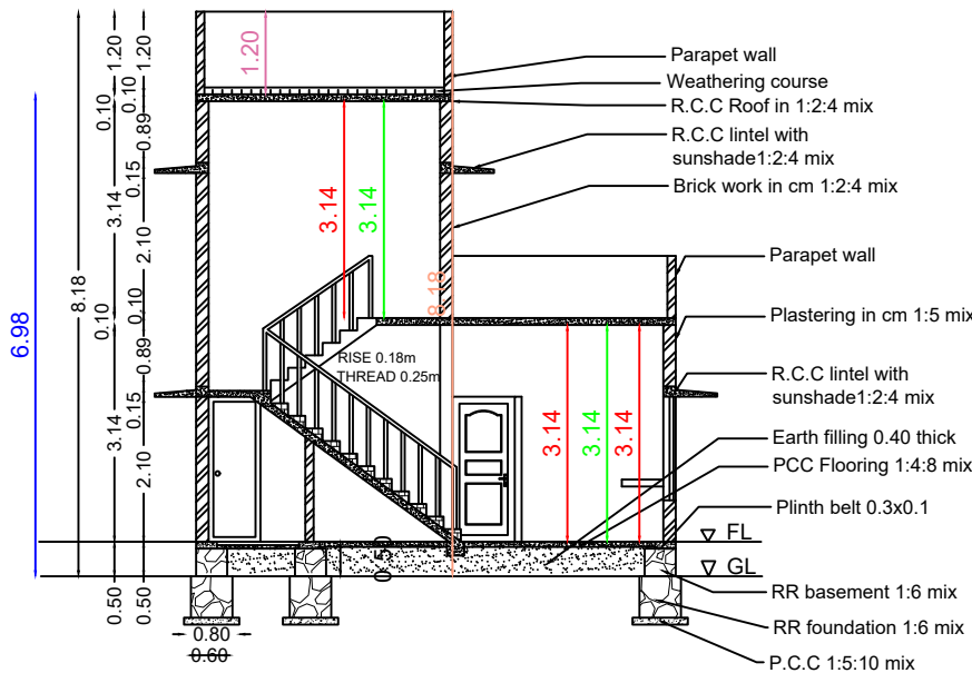
SECTION -AB
