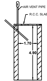
SOAK PIT
