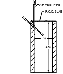
SOAK PIT
