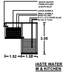
SOAK PIT
