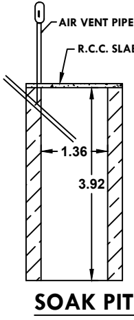
SOAK PIT
