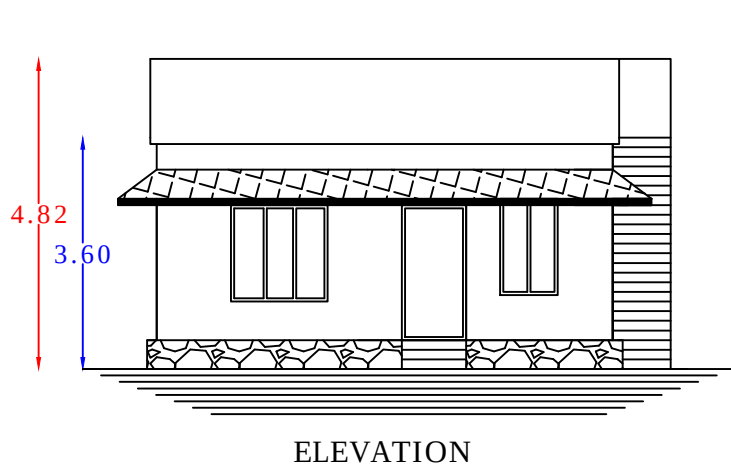
ELEVATION
